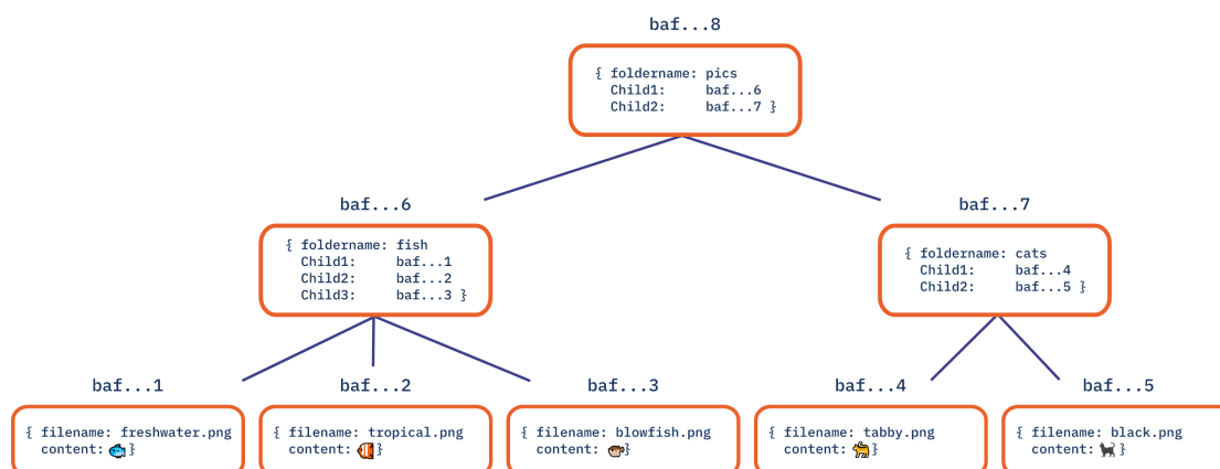
Σχήμα 2.10: Merkle DAG[16]
