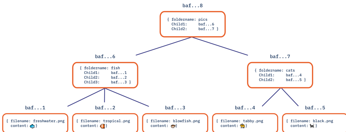
Σχήμα 2.5: Merkle DAG[14]
