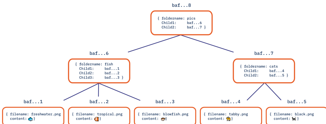
Σχήμα 2.5: Merkle DAG[15]
