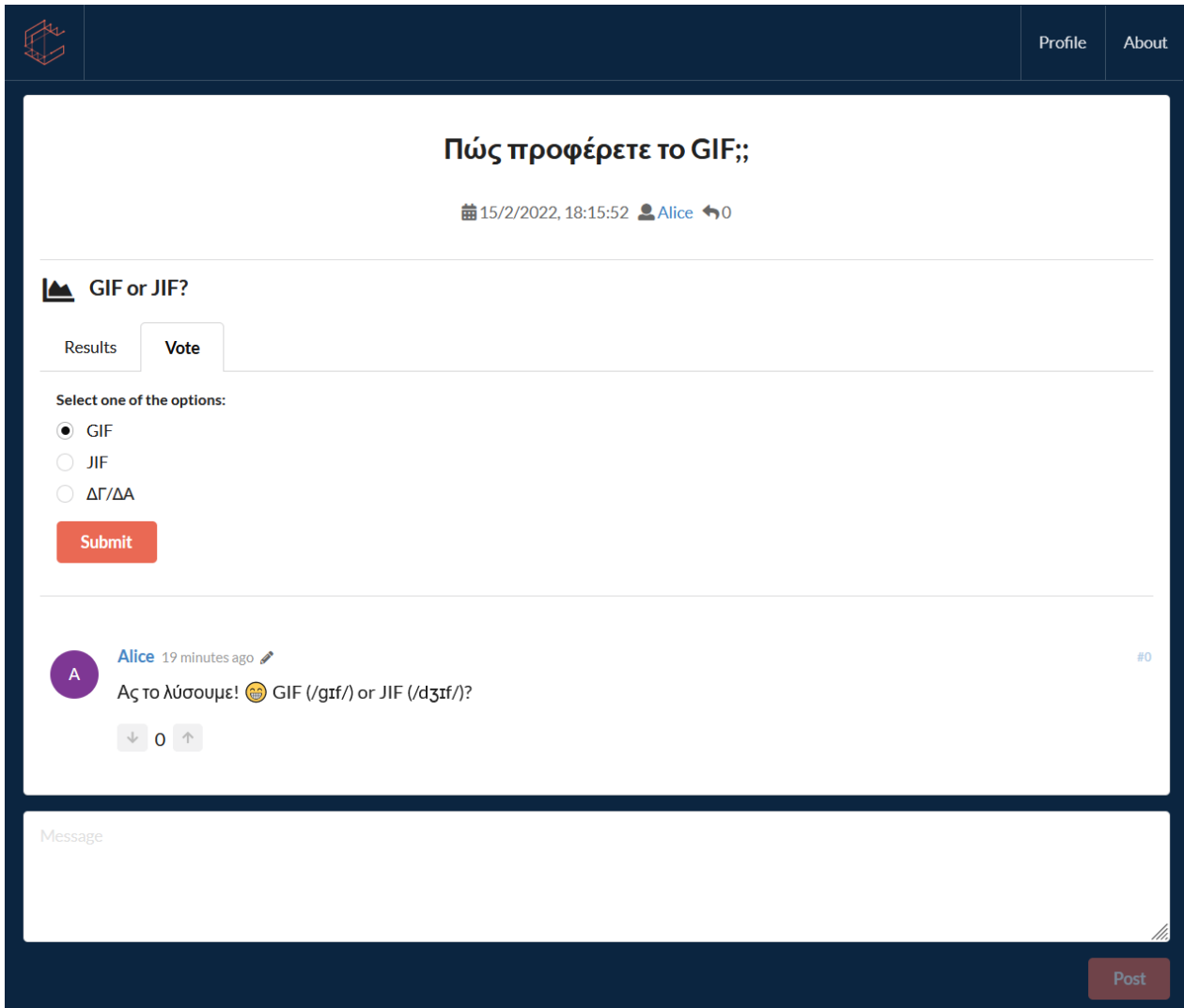
Στιγμιότυπο Corcordia A.7: Ψήφιση σε ψηφοφορία (<A A-10>)
