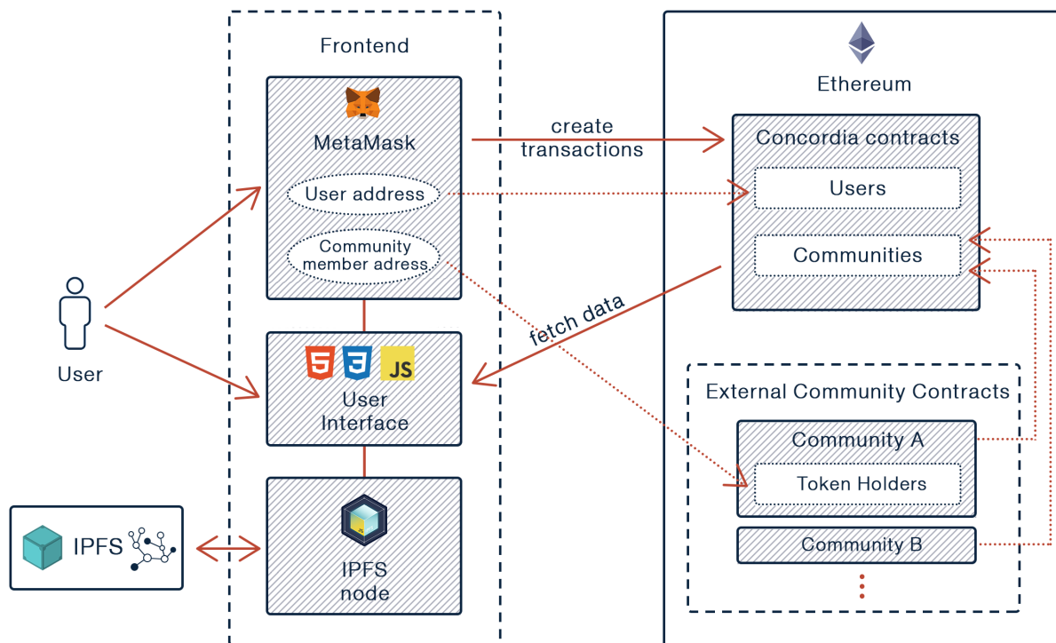
Σχήμα 3.15: Αρχιτεκτονική του συστήματος (στάδιο σχεδίασης)
