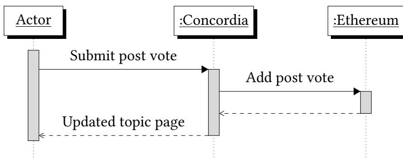
Σχήμα 3.11: Σενάριο χρήσης 8 - Διάγραμμα βασικής ροής
