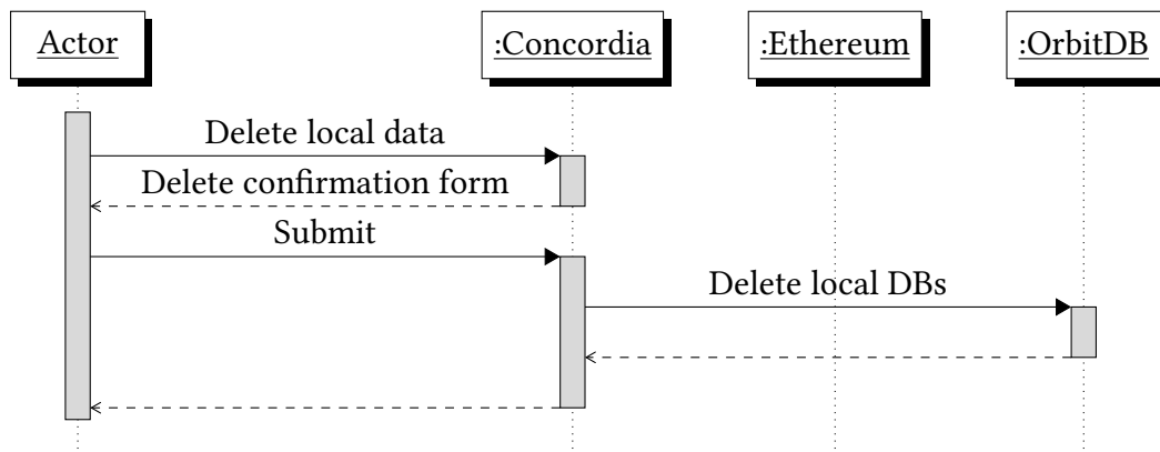
Σχήμα 3.12: Σενάριο χρήσης 9 - Διάγραμμα βασικής ροής
