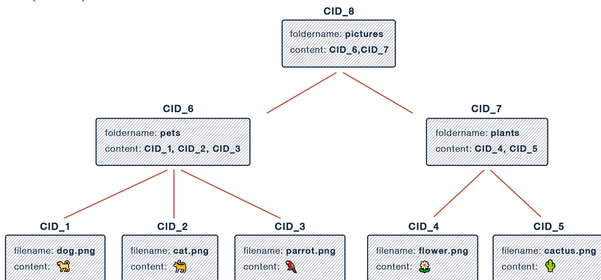
Σχήμα 2.11: Παράδειγμα Merkle DAG 14
