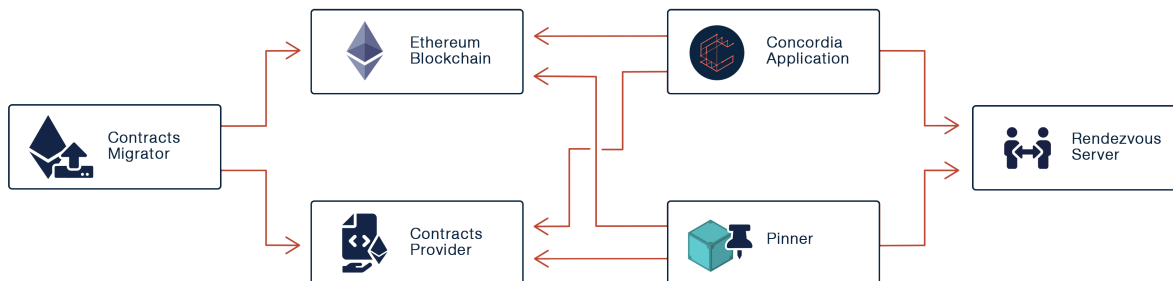
Σχήμα 4.23: Γράφος οπτικοποίησης των καναλιών επικοινωνίας των μικροϋπηρεσιών
