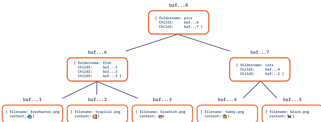
Σχήμα 2.5: Merkle DAG[15]
