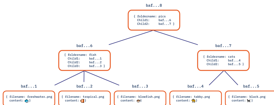
Σχήμα 2.8: Merkle DAG[17]
