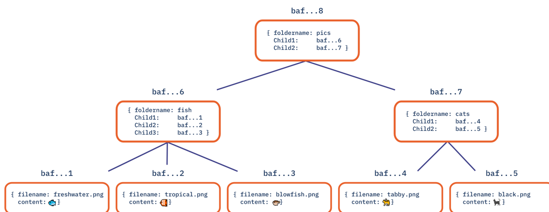
Σχήμα 2.5: Merkle DAG[17]
