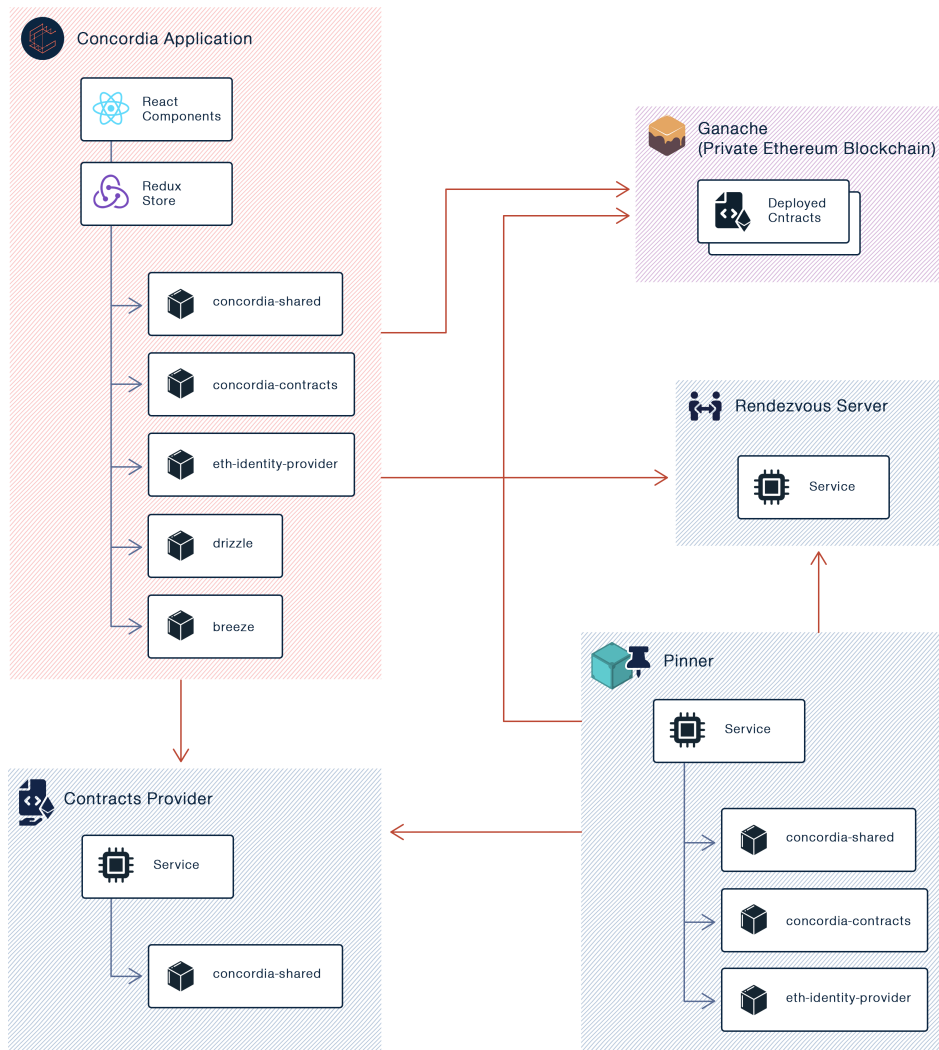
Σχήμα 4.17: Διάγραμμα αρχιτεκτονικής συστήματος
