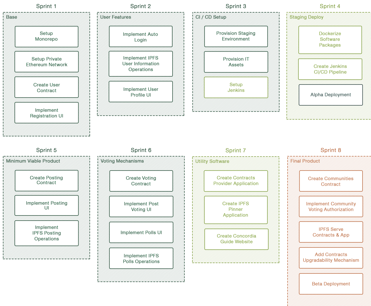
Σχήμα 4.26: Διαχωρισμός σε sprints (στάδιο υλοποίησης)
