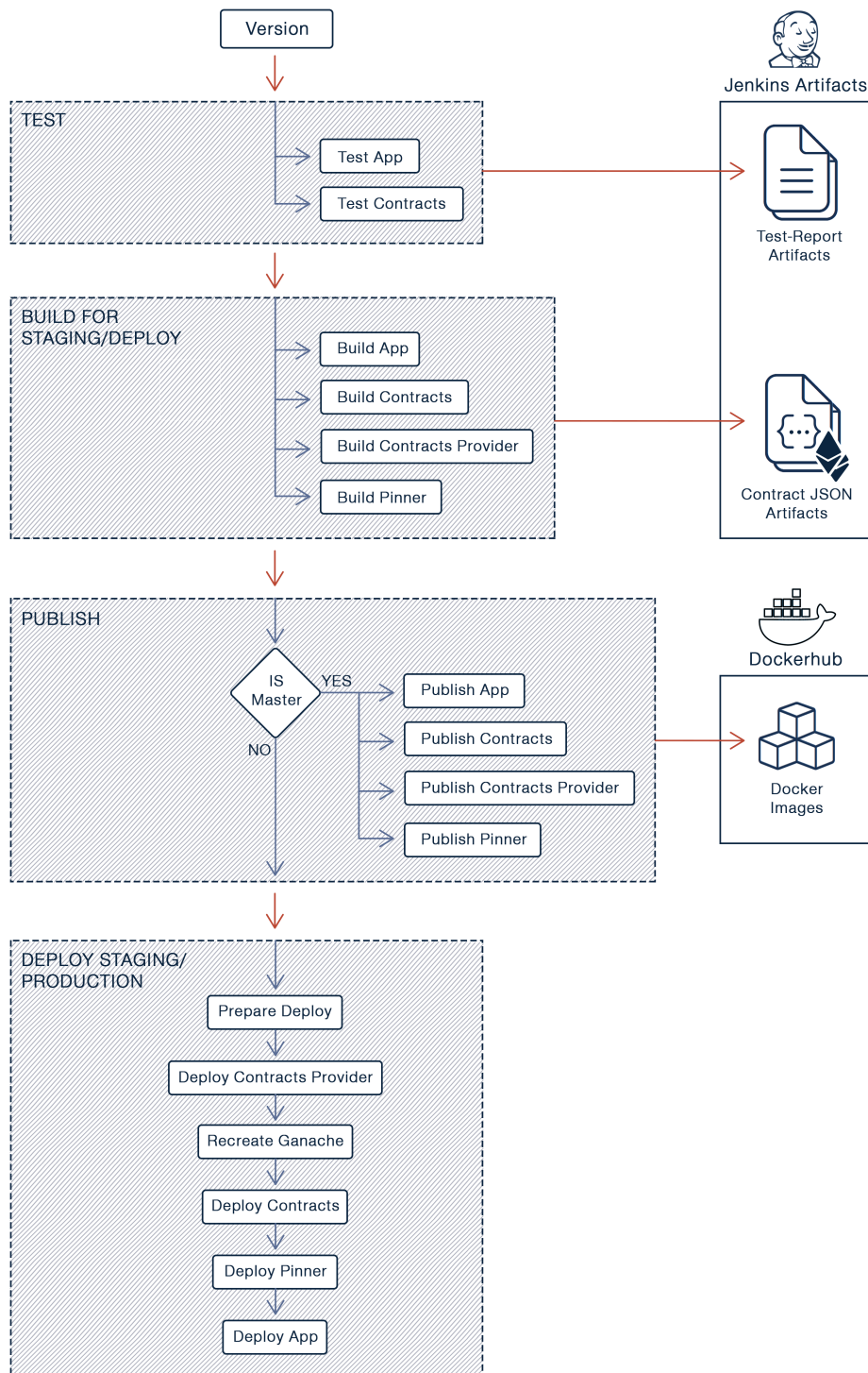
Σχήμα 4.2: Διάγραμμα ροής εργασιών Jenkins
