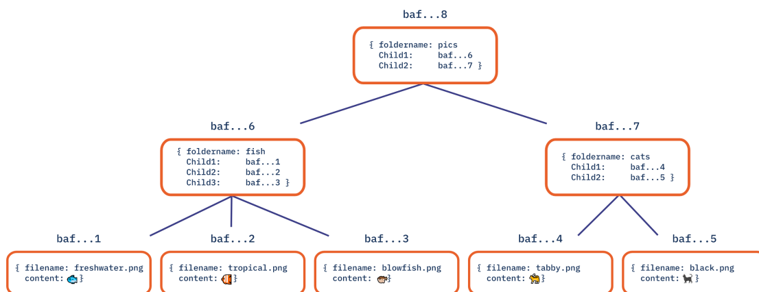
Σχήμα 2.11: Παράδειγμα Merkle DAG 13
