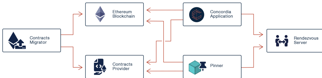
Σχήμα 4.23: Γράφος οπτικοποίησης των καναλιών επικοινωνίας των μικροϋπηρεσιών
