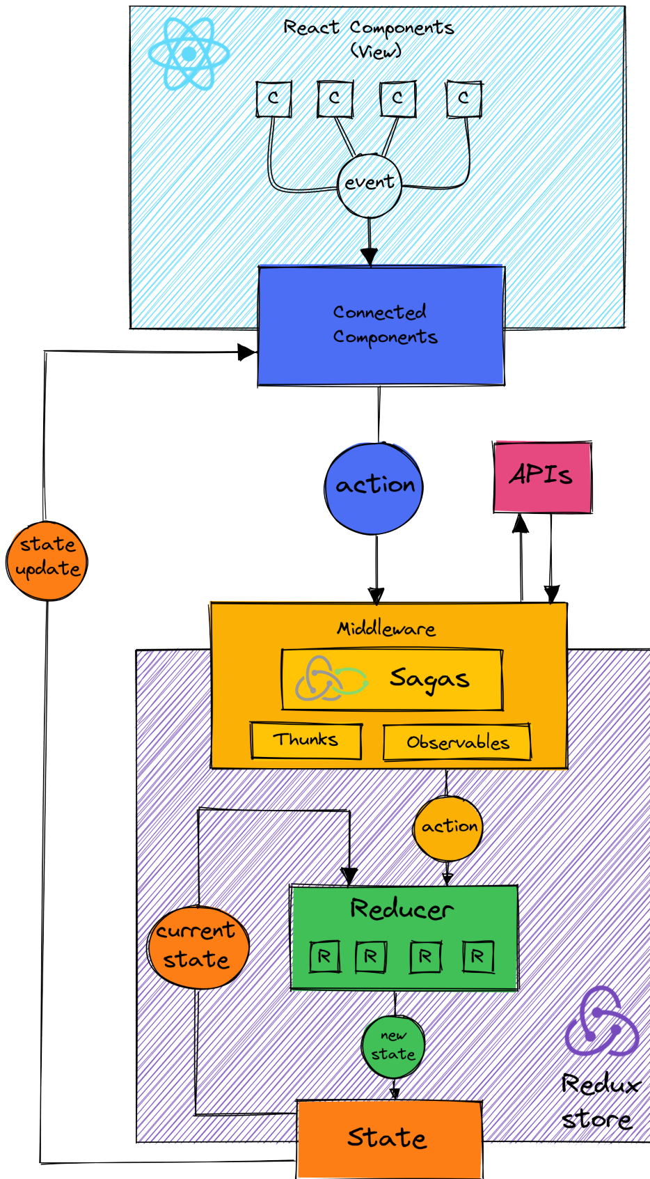
Σχήμα 4.8: Λειτουργία του Redux σε συνδυασμό με React
