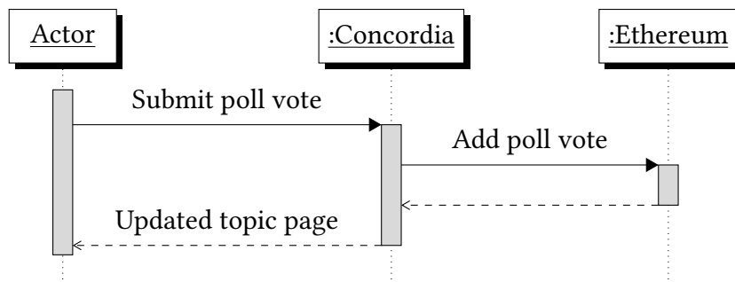
Σχήμα 3.7: Σενάριο χρήσης 5 - Διάγραμμα βασικής ροής
