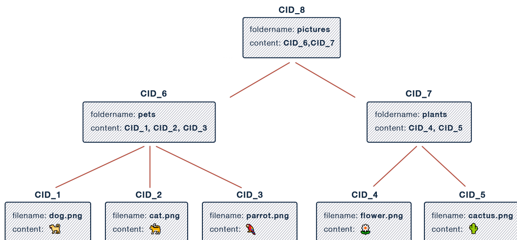
Σχήμα 2.11: Παράδειγμα Merkle DAG 14
