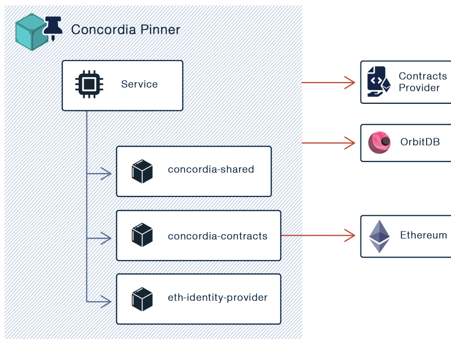
Σχήμα 4.21: Αρχιτεκτονική υπηρεσίας Concordia Pinner
