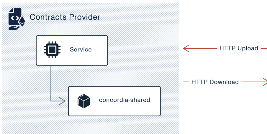
Σχήμα 4.22: Αρχιτεκτονική υπηρεσίας Concordia Contracts Provider
