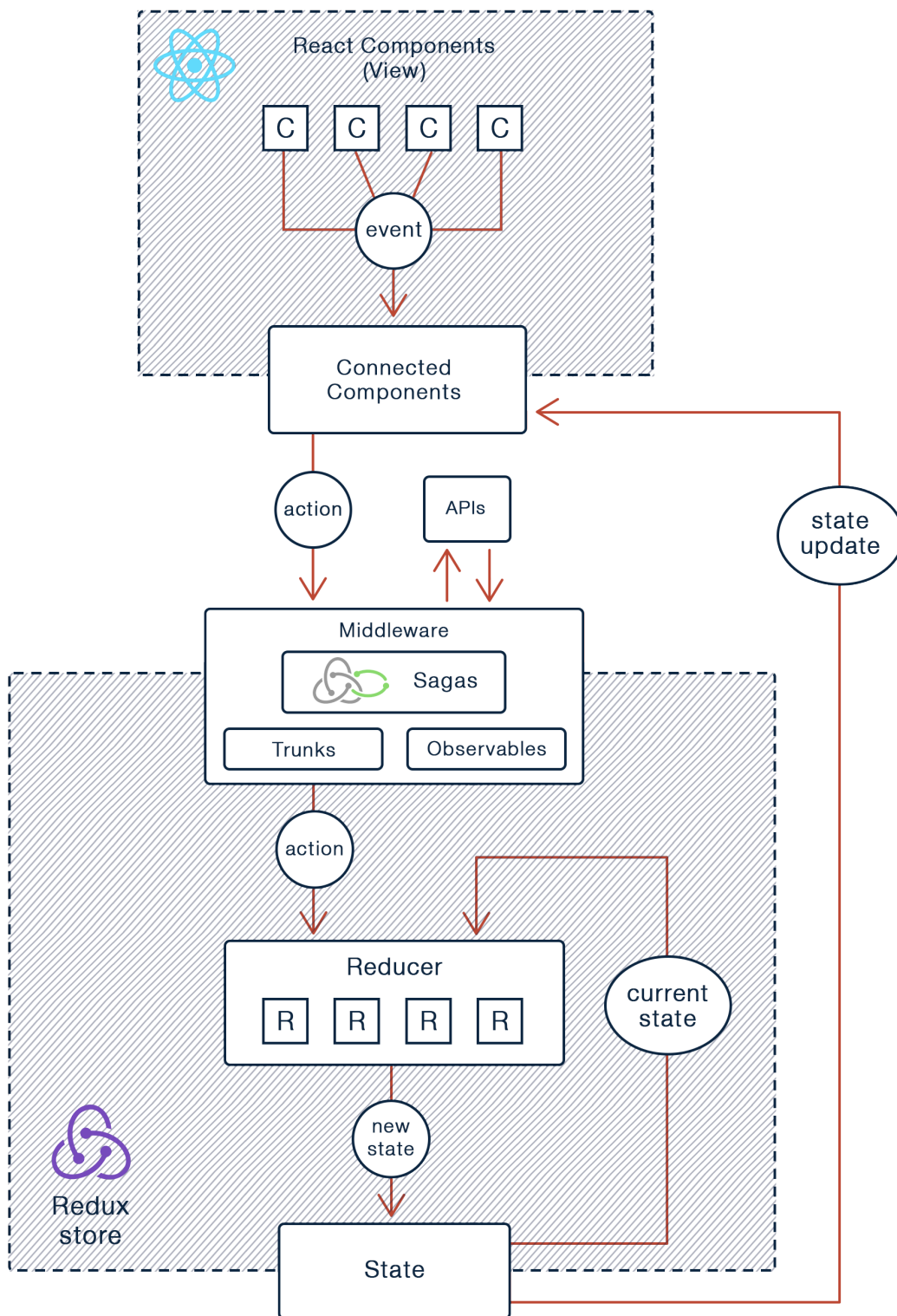
Σχήμα 4.8: Λειτουργία του Redux σε συνδυασμό με React
