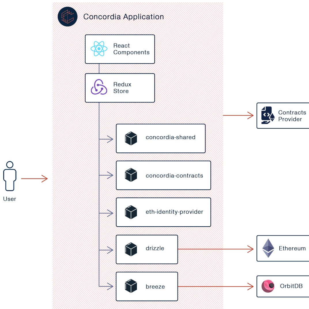
Σχήμα 4.19: Αρχιτεκτονική υπηρεσίας Concordia Application
