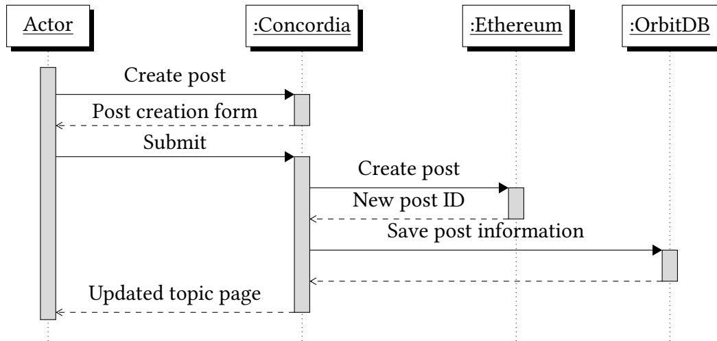
Σχήμα 3.8: Σενάριο χρήσης 5 - Διάγραμμα βασικής ροής
