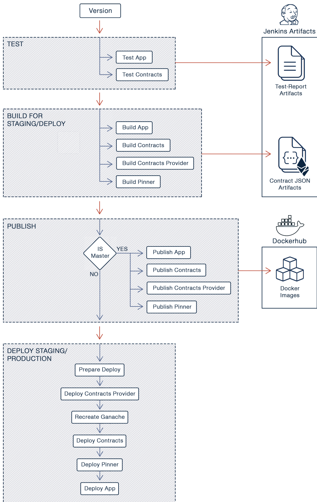
Σχήμα 4.2: Διάγραμμα ροής εργασιών Jenkins
