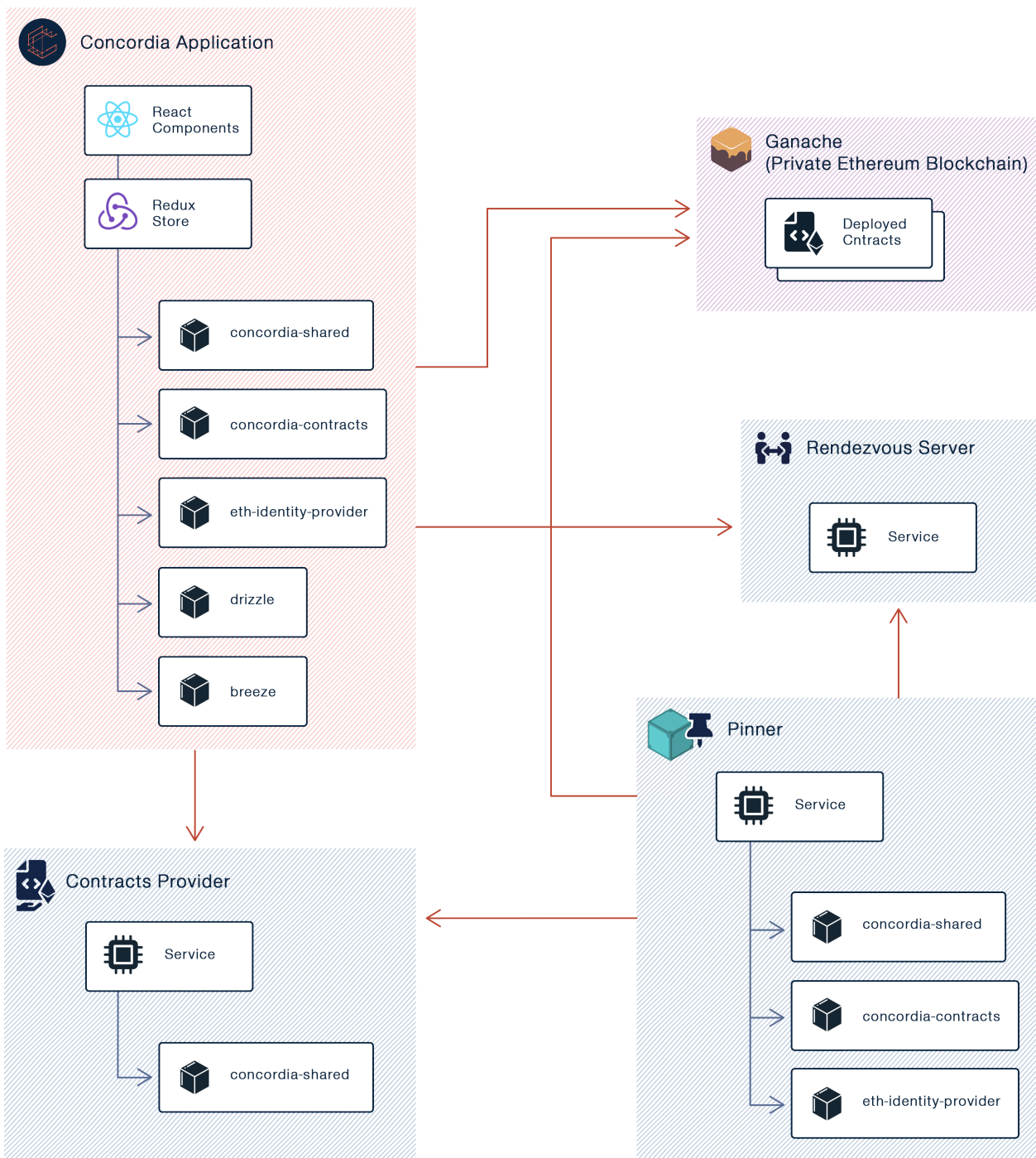
Σχήμα 4.17: Διάγραμμα αρχιτεκτονικής συστήματος
