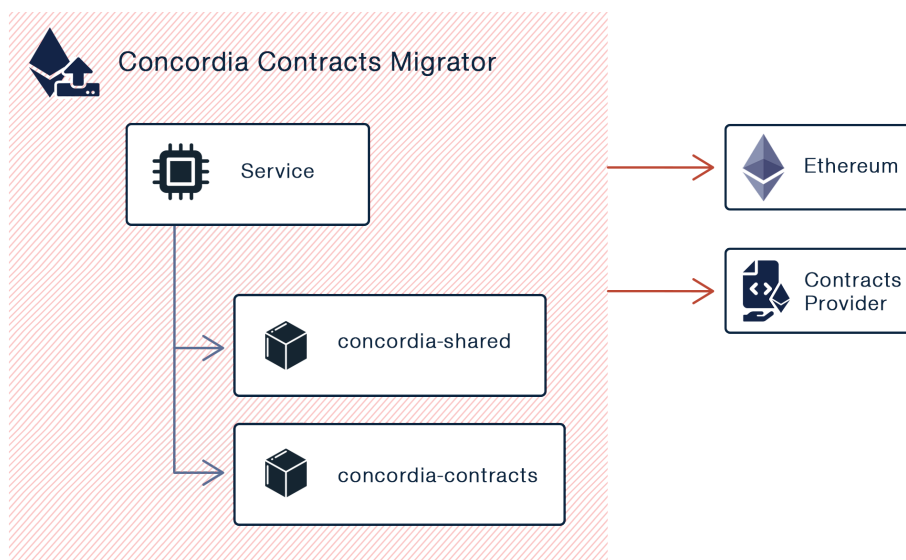
Σχήμα 4.20: Αρχιτεκτονική υπηρεσίας Concordia Contracts Migrator
