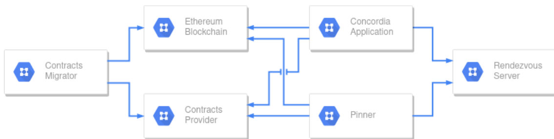
Σχήμα 4.1: Γράφος οπτικοποίησης των καναλιών επικοινωνίας των μικροϋπηρεσιών
