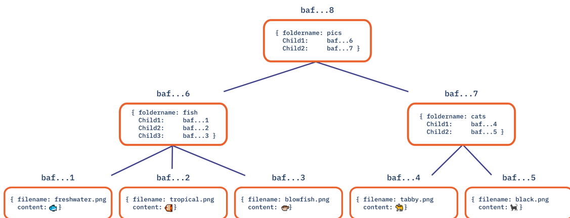
Σχήμα 2.5: Merkle DAG[8]
