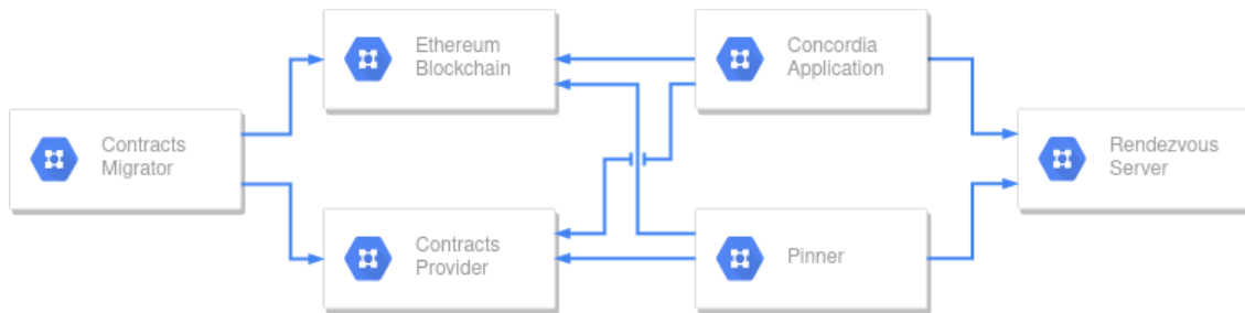
Σχήμα 4.23: Γράφος οπτικοποίησης των καναλιών επικοινωνίας των μικροϋπηρεσιών
