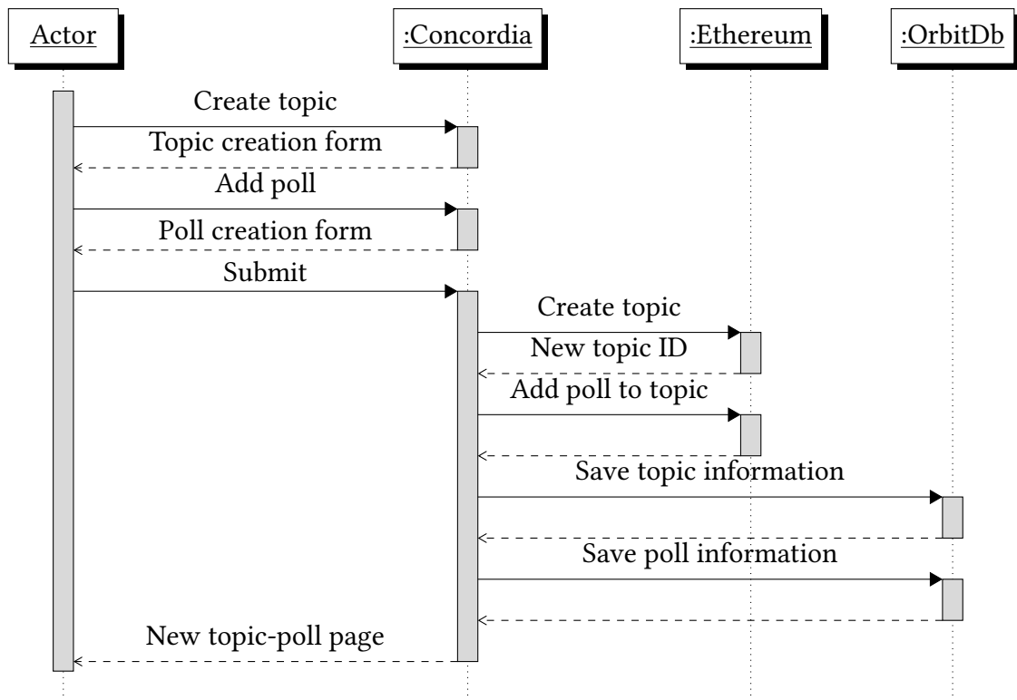
Σχήμα 3.3: Σενάριο χρήσης 2 - Διάγραμμα εναλλακτικής ροής 1
