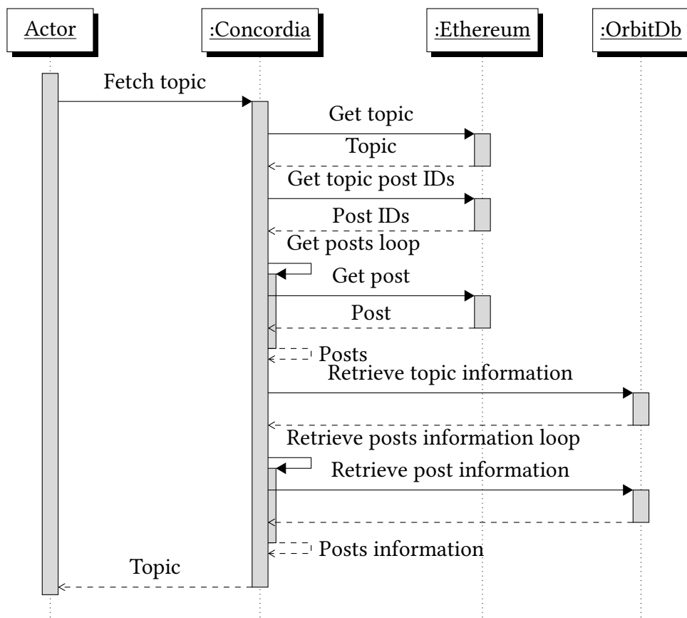
Σχήμα 3.4: Σενάριο χρήσης 3 - Διάγραμμα βασικής ροής
