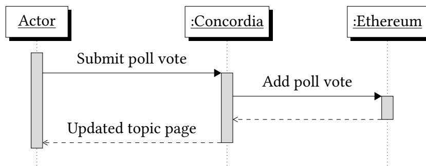
Σχήμα 3.7: Σενάριο χρήσης 5 - Διάγραμμα βασικής ροής
