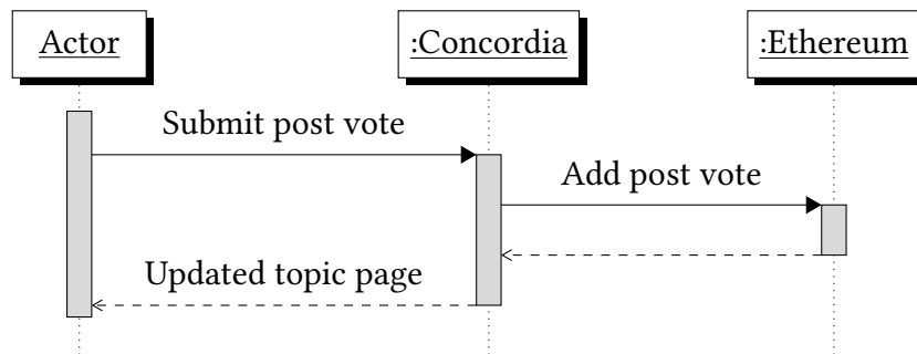
Σχήμα 3.8: Σενάριο χρήσης 6 - Διάγραμμα βασικής ροής
