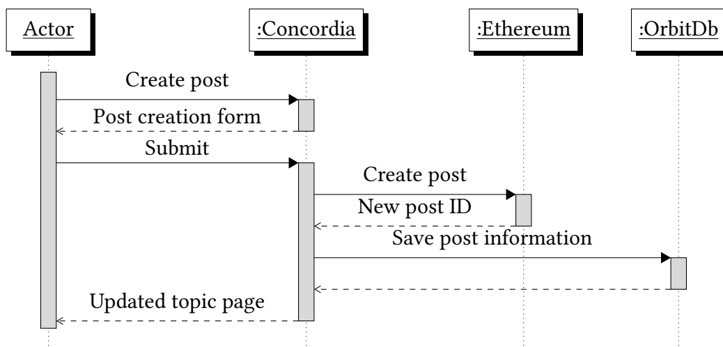
Σχήμα 3.6: Σενάριο χρήσης 4 - Διάγραμμα βασικής ροής
