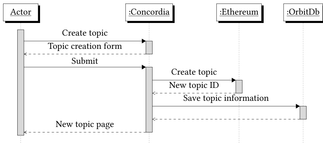
Σχήμα 3.2: Σενάριο χρήσης 2 - Διάγραμμα βασικής ροής
