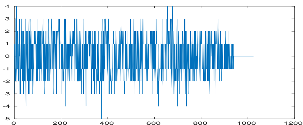
Σχήμα 10: Κβαντισμένοι συντελεστές
