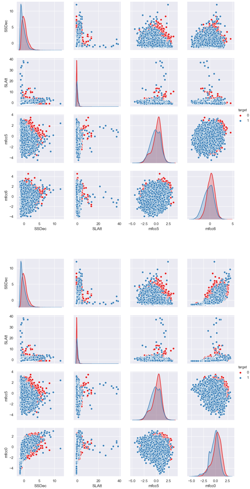
Σχήμα 1: Αποτελεσματικότητα χαρακτηριστικών στον διαχωρισμό των κλάσεων
